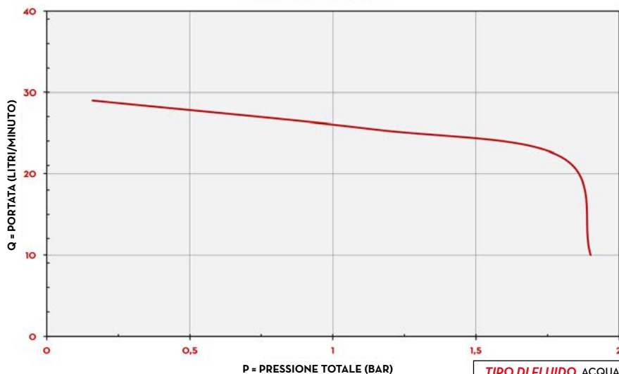
PISTOLA AUTOMATICA
