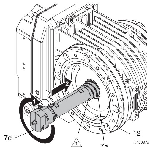
FIG. 17 : Insérer l'outil de graissage du rotor
