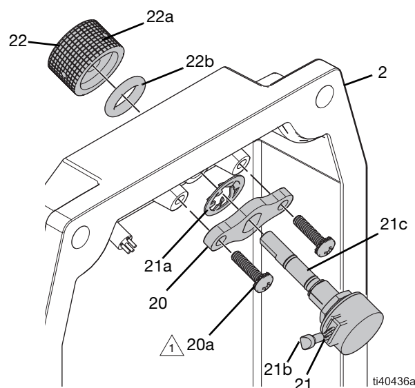
FIG. 10 : Assemblage du bouton de commande
