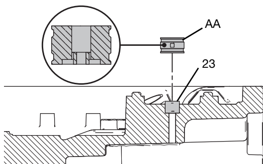
Fig. 7: Douille de pressage sur le roulement du moteur
