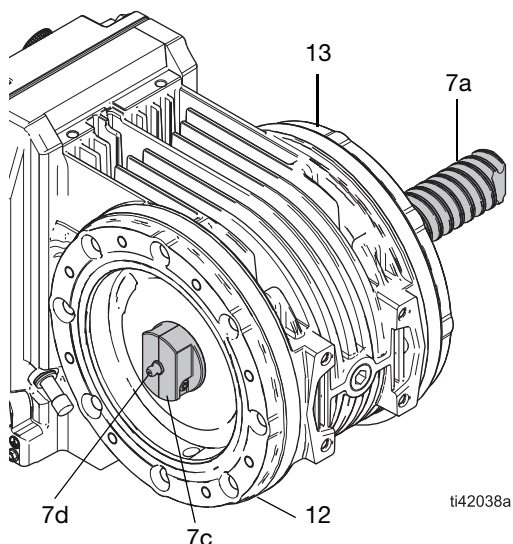
Fig. 18 : Outil de graissage du rotor
