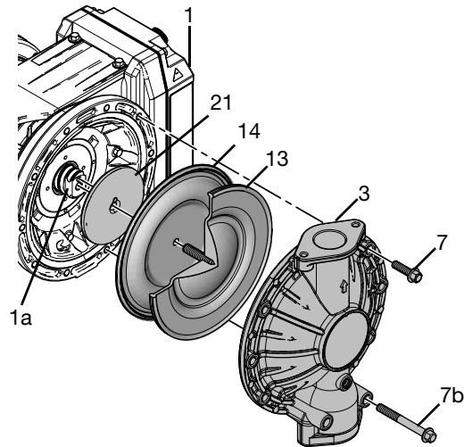
ABB. 22: Umgossene Membranen
