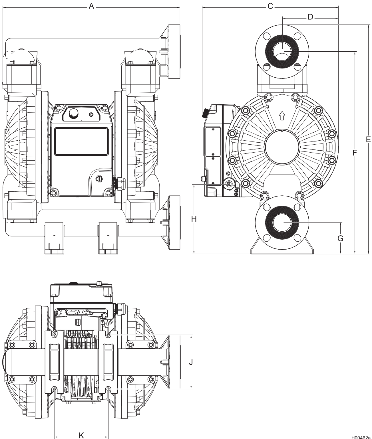
ABB. 31: Abmessungsdiagramm für i120-Kugelmodelle mit materialberührtem Abschnitt aus Kunststoff
