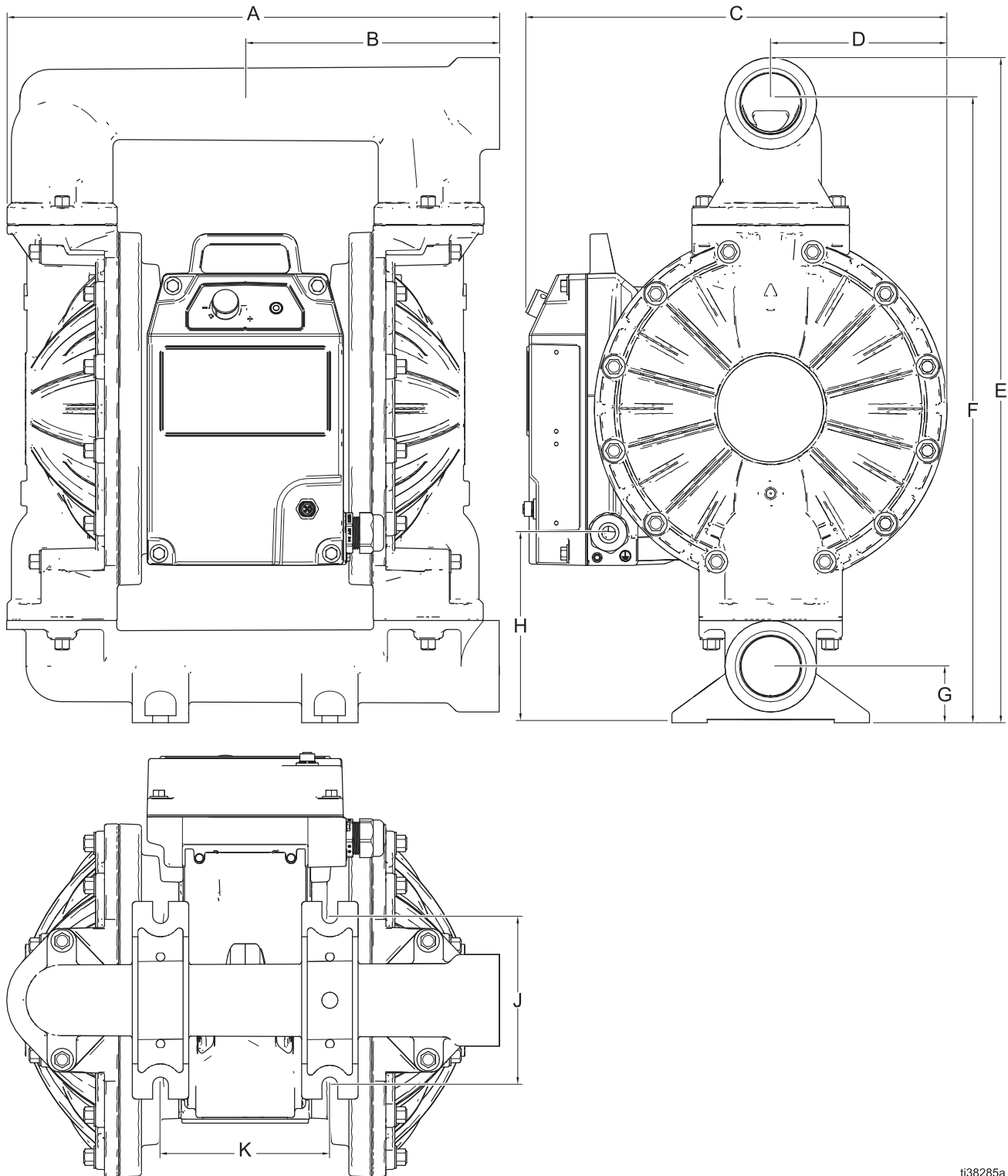
ABB. 30: Abmessungsdiagramm für i120 (QTE) Kugelmodelle mit materialberührtem Abschnitt aus Metall
