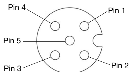
ABB. 14: M12, 5-poliger Stecker für Modelle an gewöhnlichen Standorten
