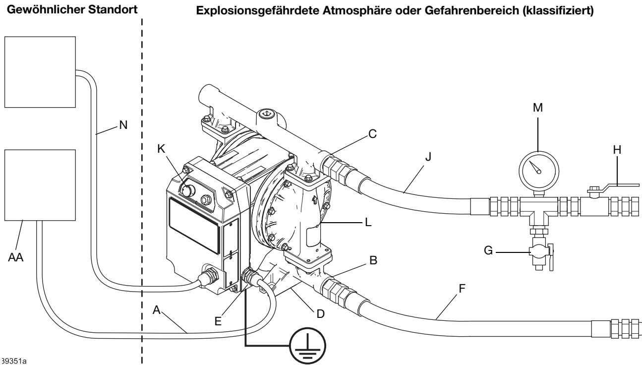
ABB. 4: Typische Installation für Modelle in explosiven Atmosphären oder Gefahrenbereichen (klassifiziert) (fest verdrahtet für permanenten Anschluss) (Modell i30 (QTC) abgebildet)
