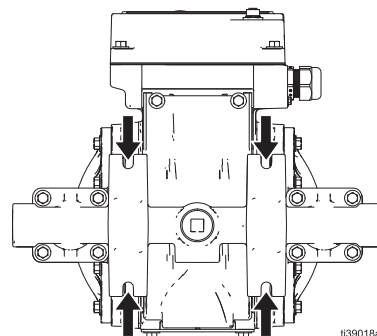
ABB. 7: Montagebohrungen
