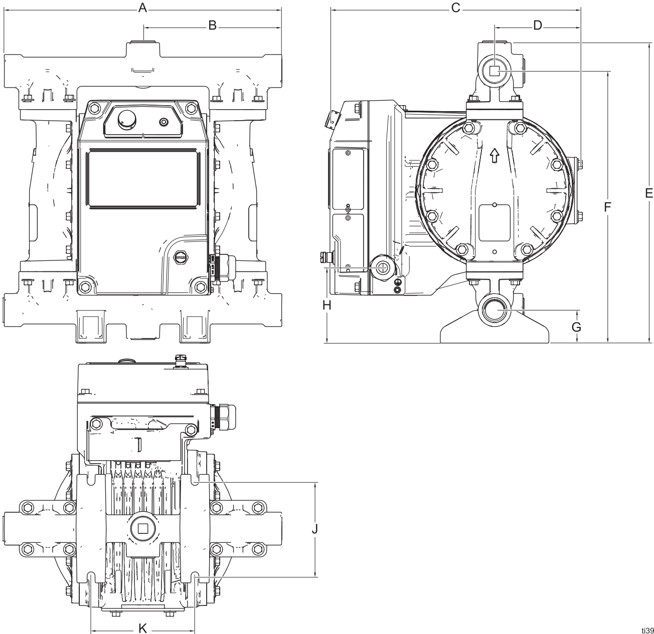
ABB. 25: Abmessungsdiagramm für i30 (QTC) mit materialberührtem Abschnitt aus Metall
