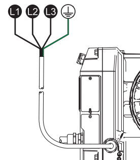
ABB. 13: Verdrahtung für 3-phasige Modelle
