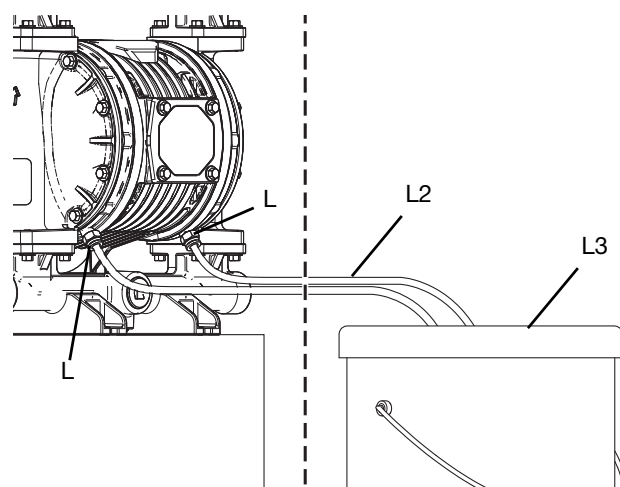
ABB. 9: Typische Installation von Materiallekkleitungen (gewöhnliche Standorte)
