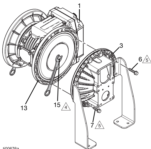
ABB. 21: Standard-Membranen festziehen
