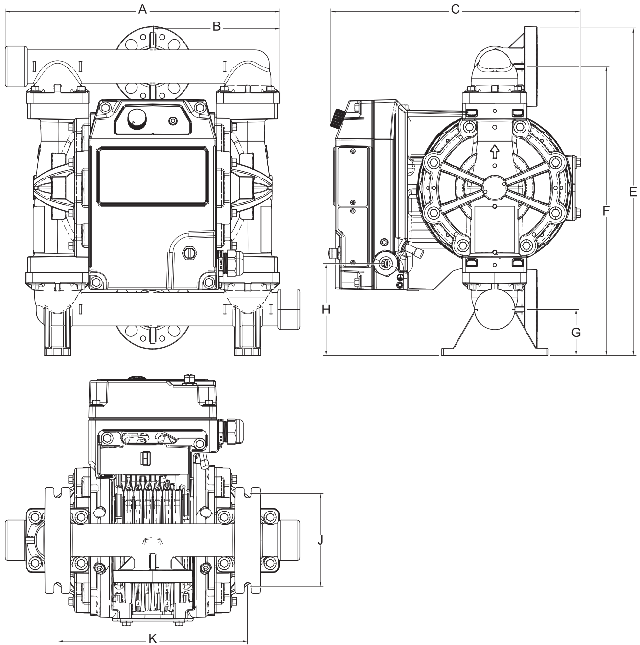
ABB. 27: Abmessungsdiagramm für i30 (QTC) mit materialberührtem Abschnitt aus Kunststoff (Mittelflansch)
