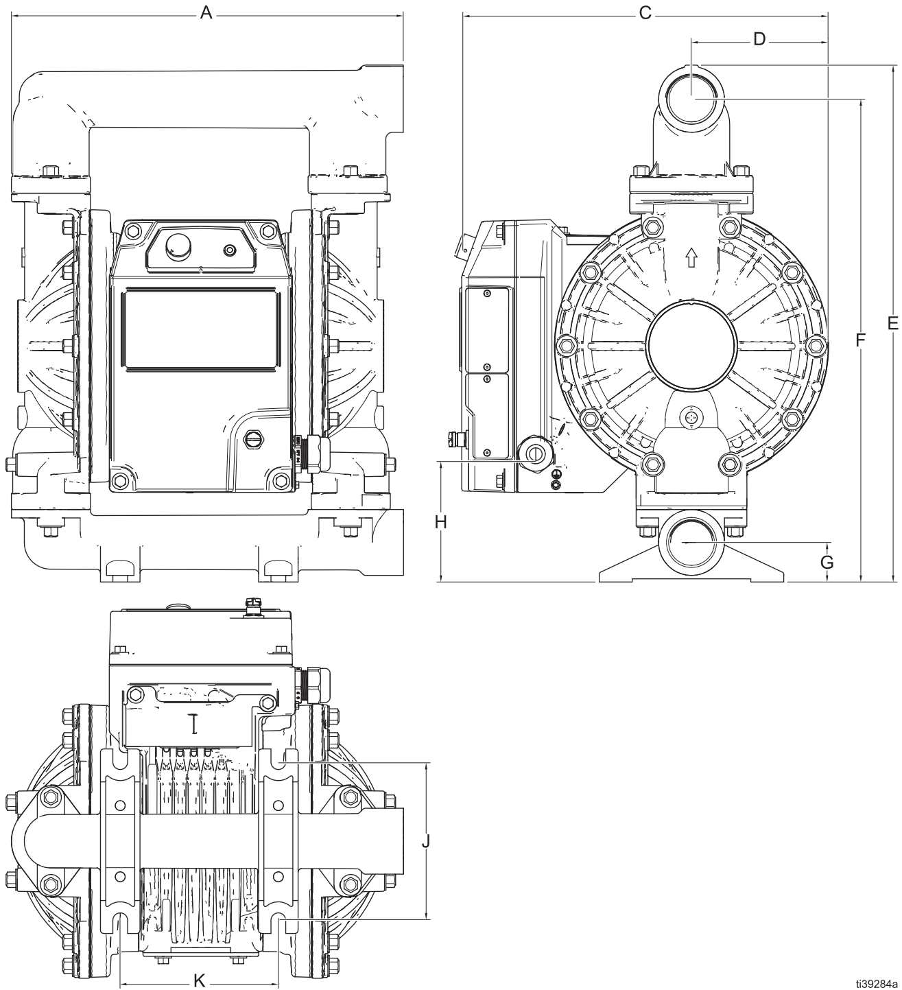
ABB. 28: Abmessungsdiagramm für i80 (QTD) Modell mit materialberührtem Abschnitt aus Metall
