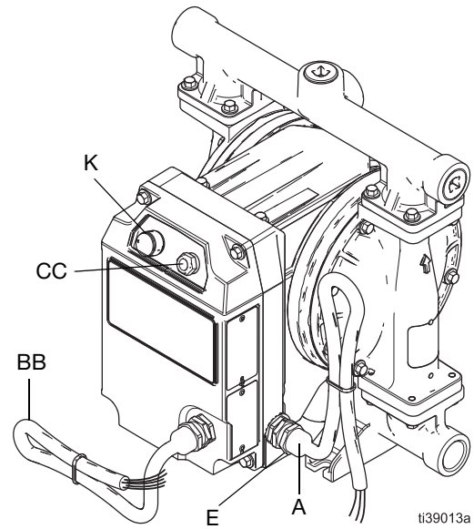
ABB. 2: Modell für explosive Atmosphären oder Gefahrenbereiche (klassifiziert) (Modell i30 (QTC) abgebildet)
