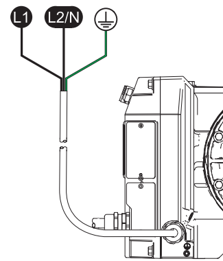
ABB. 12: Verdrahtung für einphasige Modelle
