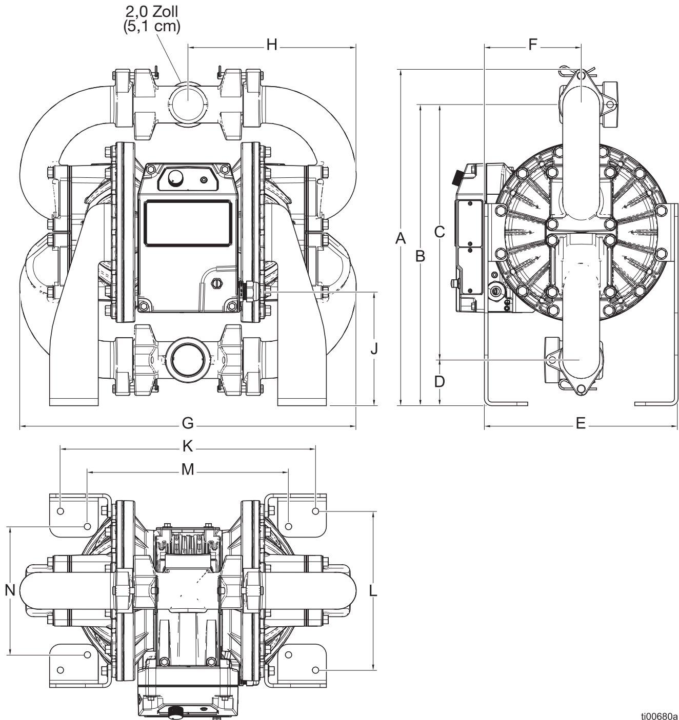
ABB. 32: Abmessungsdiagramm für i120 (QTE) Klappenmodelle mit materialberührtem Abschnitt aus Metall
