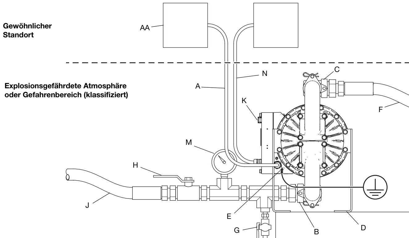
ABB. 6: Typische Installation für i120 (QTE) Klappenmodelle in explosiven Atmosphären oder gefährlichen (klassifizierten) Bereichen (fest verdrahtet für permanenten Anschluss)
