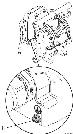
ABB. 10: Erdungsbefestigung des Geräts
