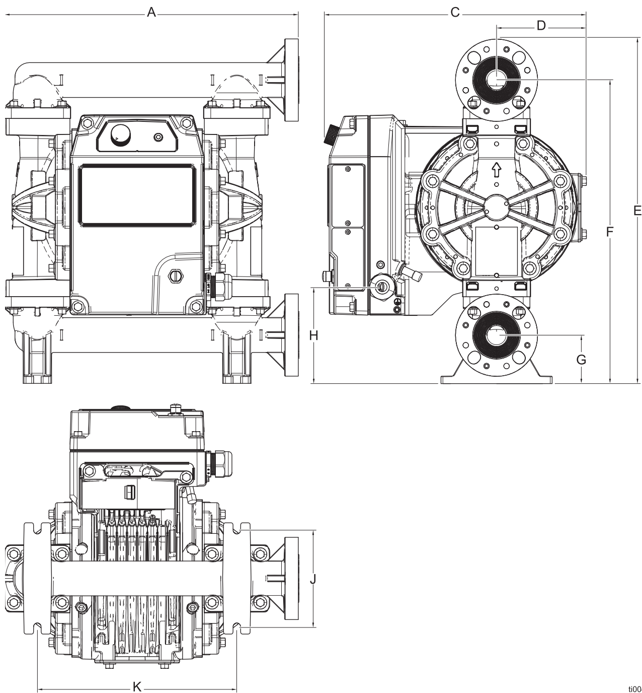
ABB. 26: Abmessungsdiagramm für i30 (QTC) mit materialberührtem Abschnitt aus Kunststoff, Endflansch
