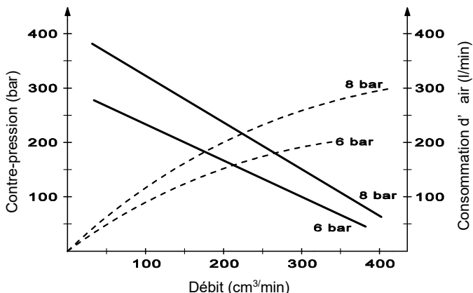
Diagramme de performances : (Graisse polyvalente NLGI, classe 2 à 20°C environ)
